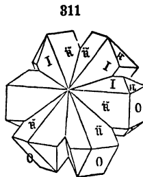
Staurolite.
